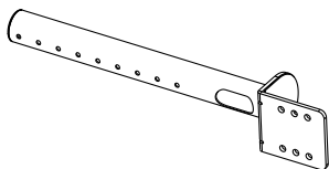
(1) Tubo di supporto da 48mm-a (1) 48mm Tube Support-a
