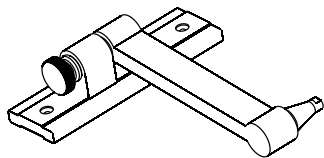
(1) Placca a muro-a (1) Wall Plate-a
